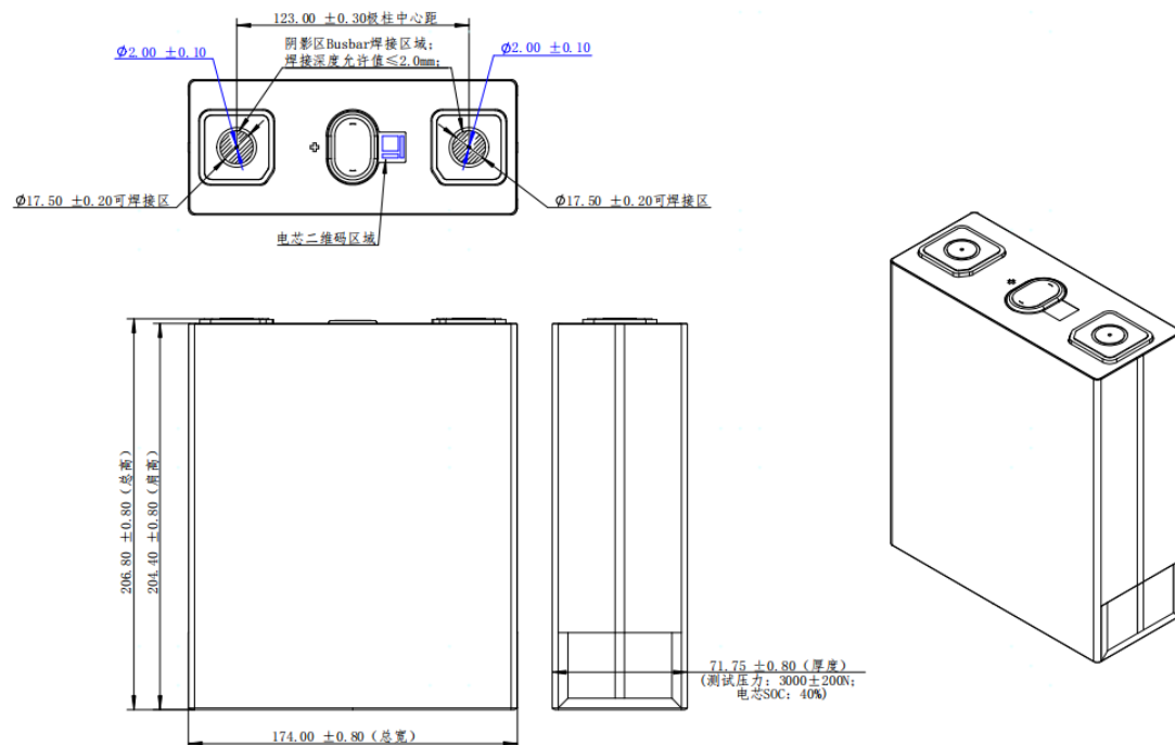
图 7.1 电池尺寸/mm
